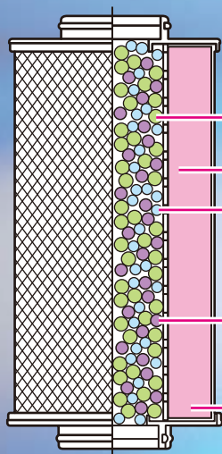
【カートリッジ断面図】
